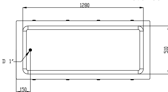
Boven aanzicht
