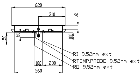
Zij aanzicht
