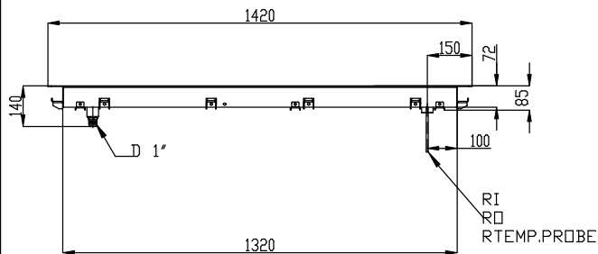
Zij aanzicht
